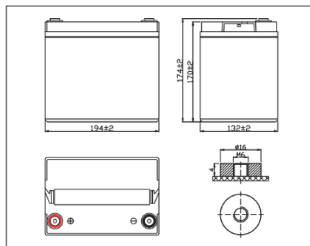
Клеммы T1
